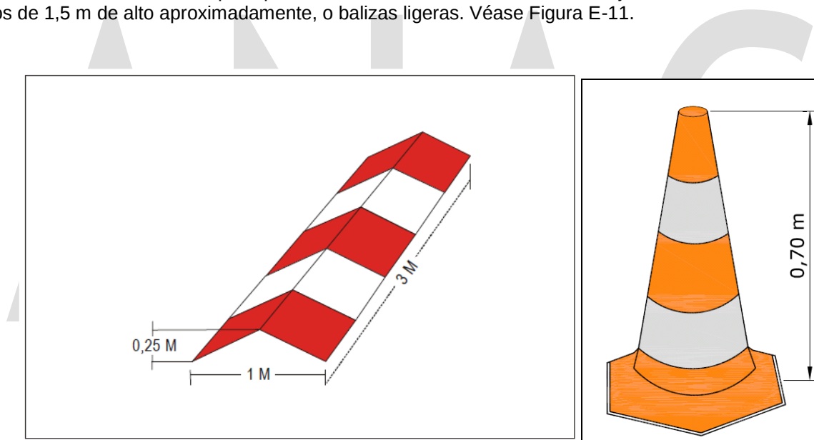
Figura E-11. Ejemplos de balizas y balizas de borde de pistas cubiertas de nieve
