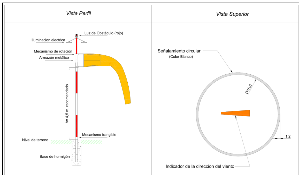
Figura E-1 Ejemplo del indicador de la dirección del viento
