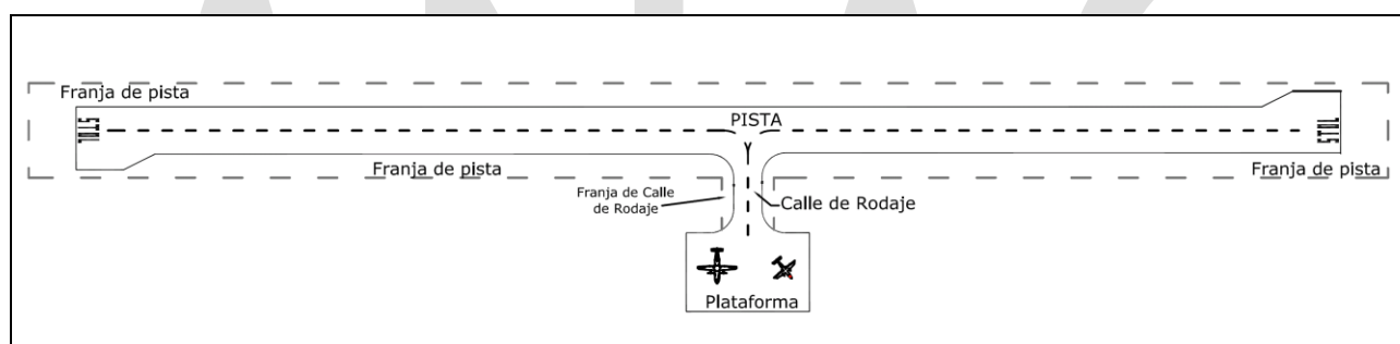
Figura C-1: Configuración básica de un aeródromo STOL
